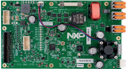
俯视图
