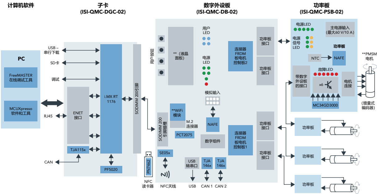
子卡 (ISI-QMC-DGC-02)
